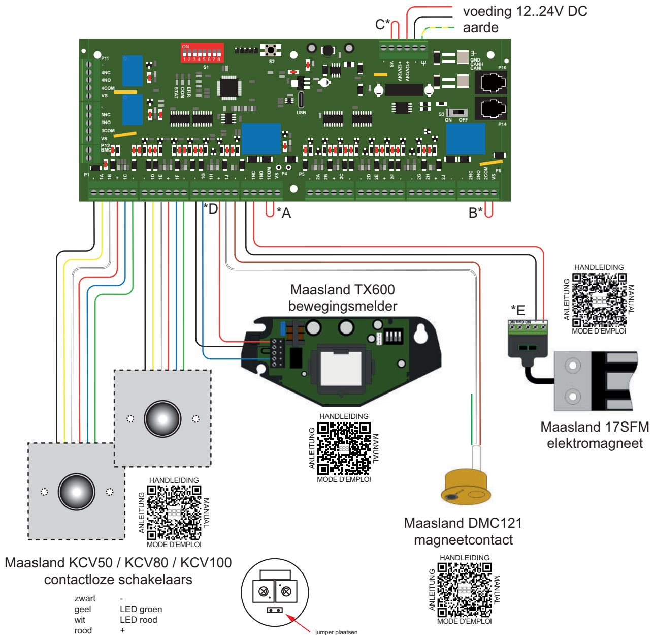
Tekening 7 Sluis met personendetector en privacy schakeling
