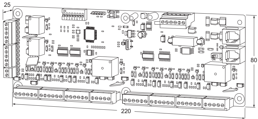
Tekening 23 Afmetingen
