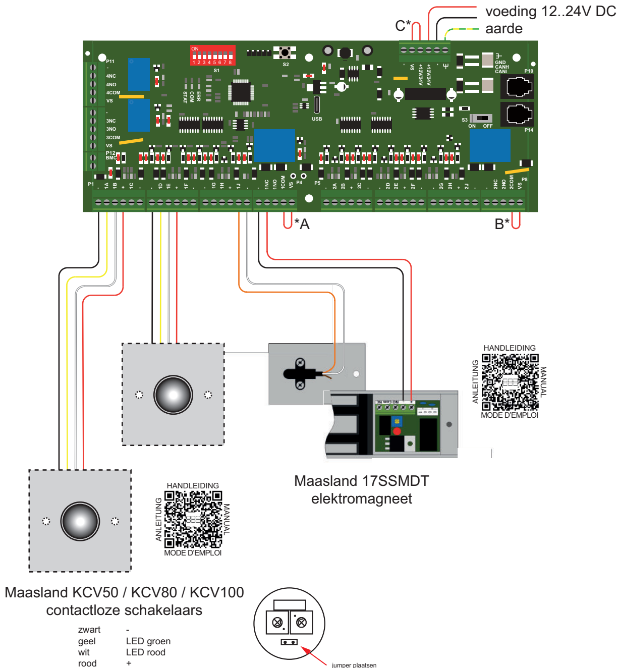
Tekening 4 Sluis - Deuren standaard ontgrendeld
