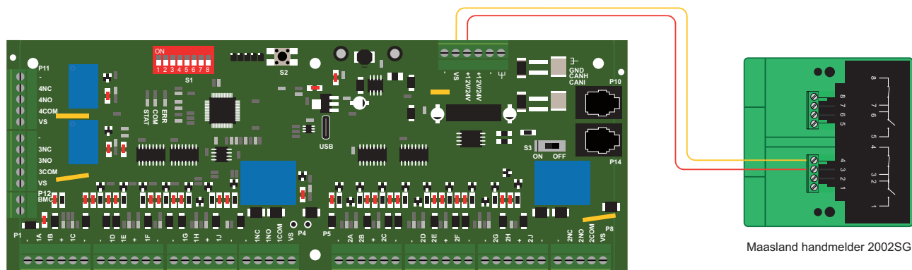
Tekening 11 Een handmelder (zonder signalering) per controller
