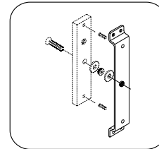
Montagesteun ankerplaat (voor model 17SFM).
